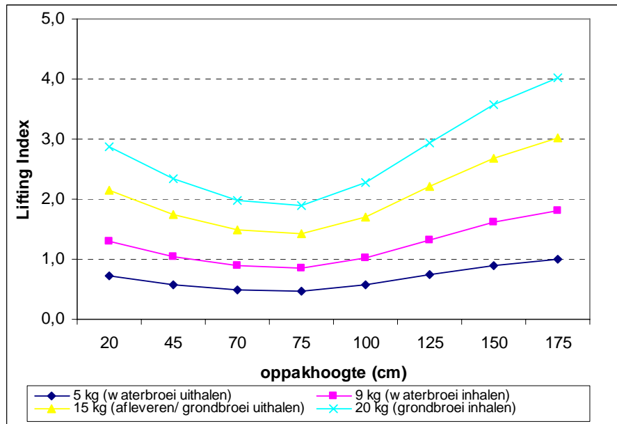
Figuur B Relatie tussen oppakhoogte en Lifting Index bij het tillen van 40x60 cm fust met verschillende in de praktijk voorkomende gewichten van of naar een hoogte van 75 cm.
