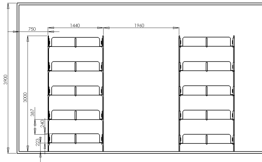
Fig 2 A en B. Standaard teeltruimte met bedden in een champignonbedrijf (ter vereenvoudiging is de klimaatinstallatie weggelaten).
